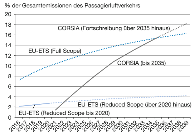
Abbildung 4 Emissionsminderung
